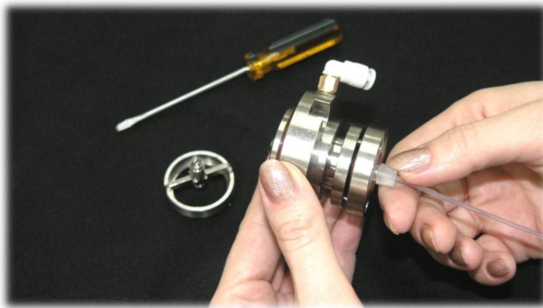
Рис. 76. Снятие капилляра
